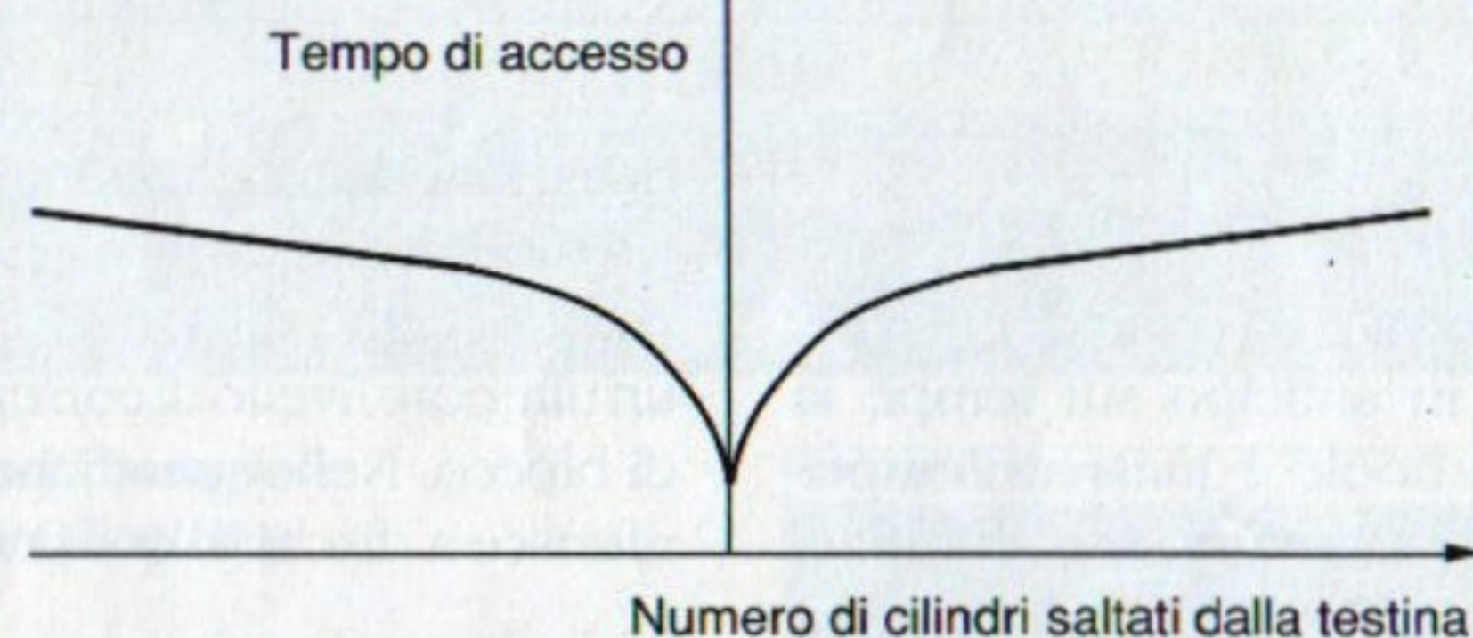
Grafici del tempo di posizionamento della testina in funzione dello spostamento radiale in un lettore di CD-ROM e in un hard disk voice-coil che non usa la tecnica "zone recording". L'origine delle ascisse indica la posizione corrente.
