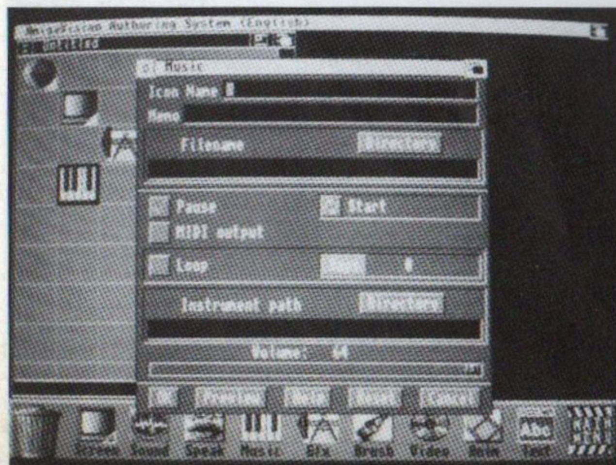
Tutte le possibilità dell'icona «Music»: si noti in particolare l'opzione «MIDI Output».
