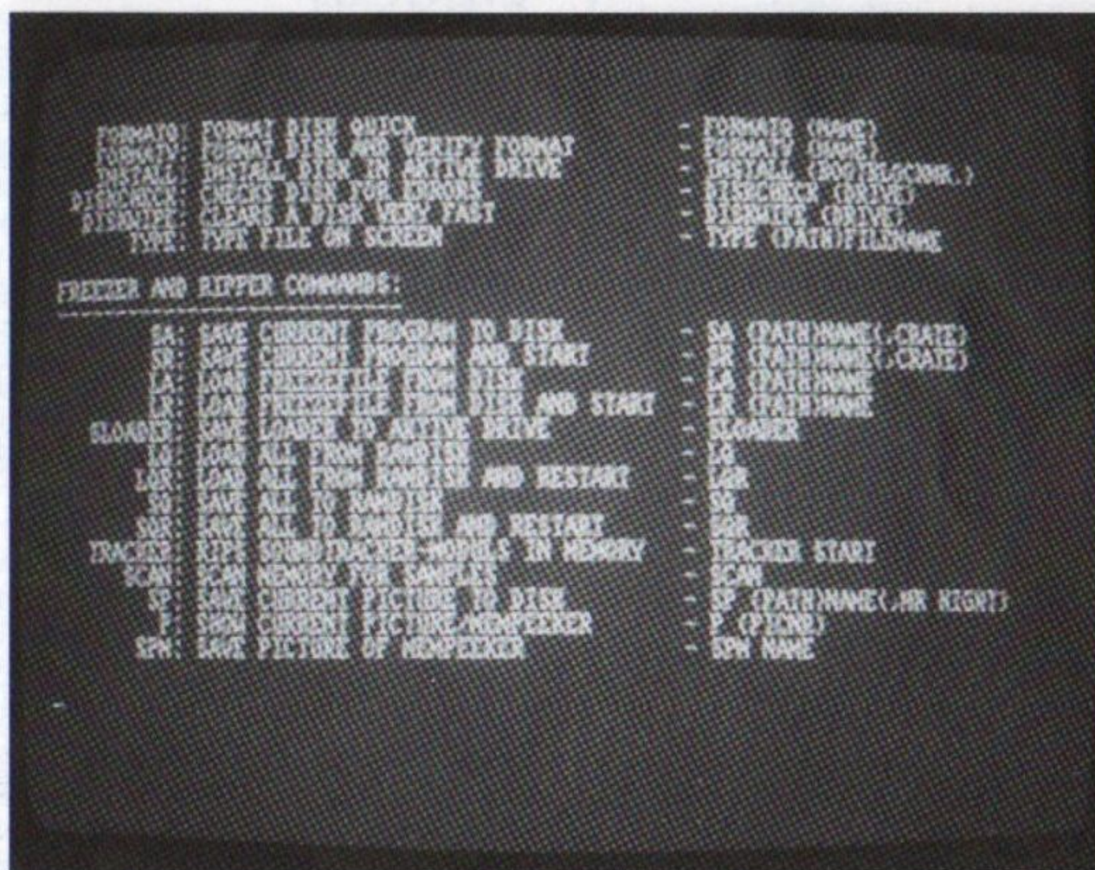
I comandi relativi alle funzioni «Freezer» e «Ripper» per la protezione di programmi e musica.
