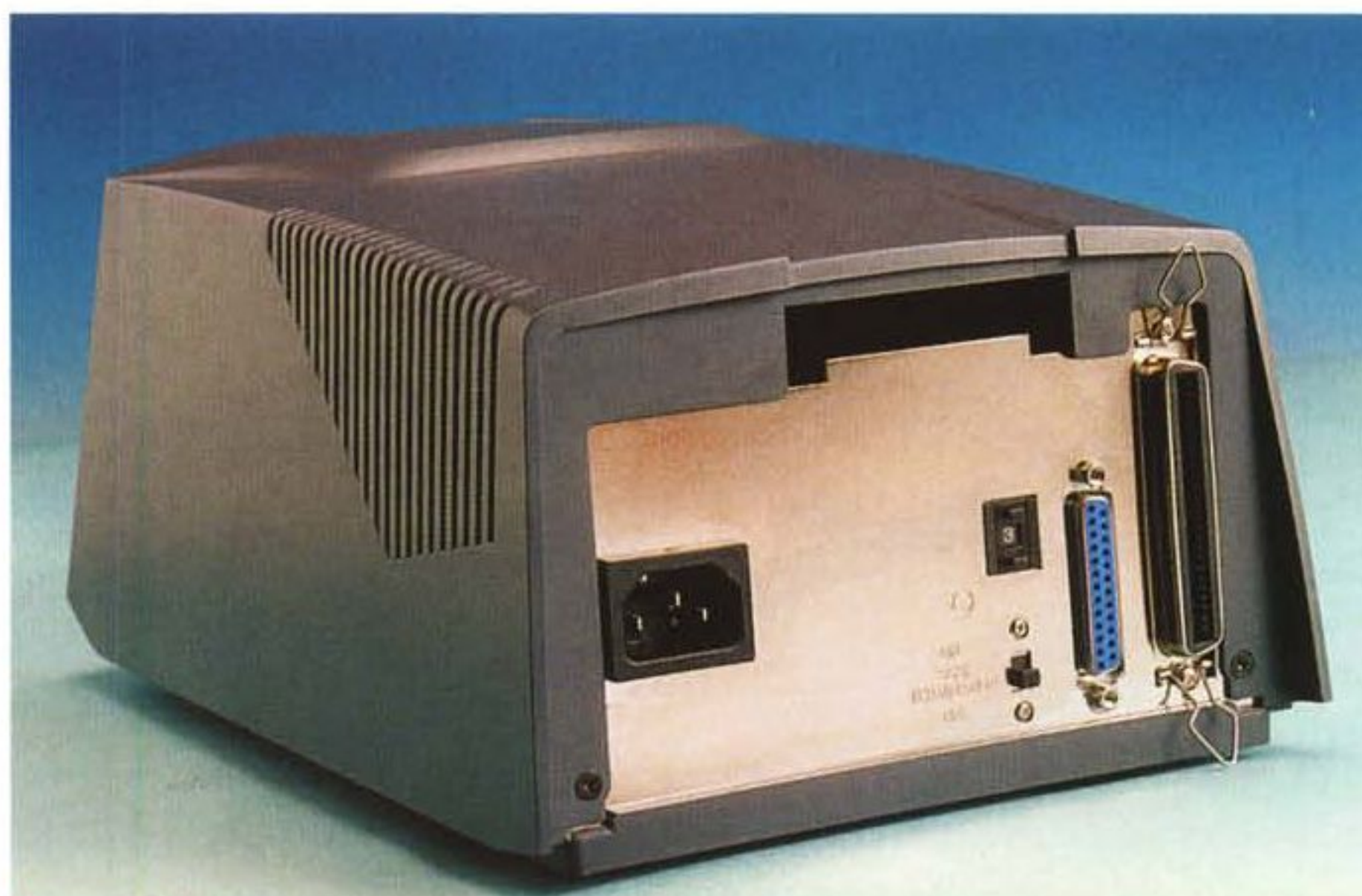
Pannello posteriore dello scanner: in evidenza le solite connessioni SCSI, il selettore dell'ID, il connettore di alimentazione e il pulsante per l'inserimento della terminazione. La fessura in alto serve per far fuoriuscire il caricatore.
