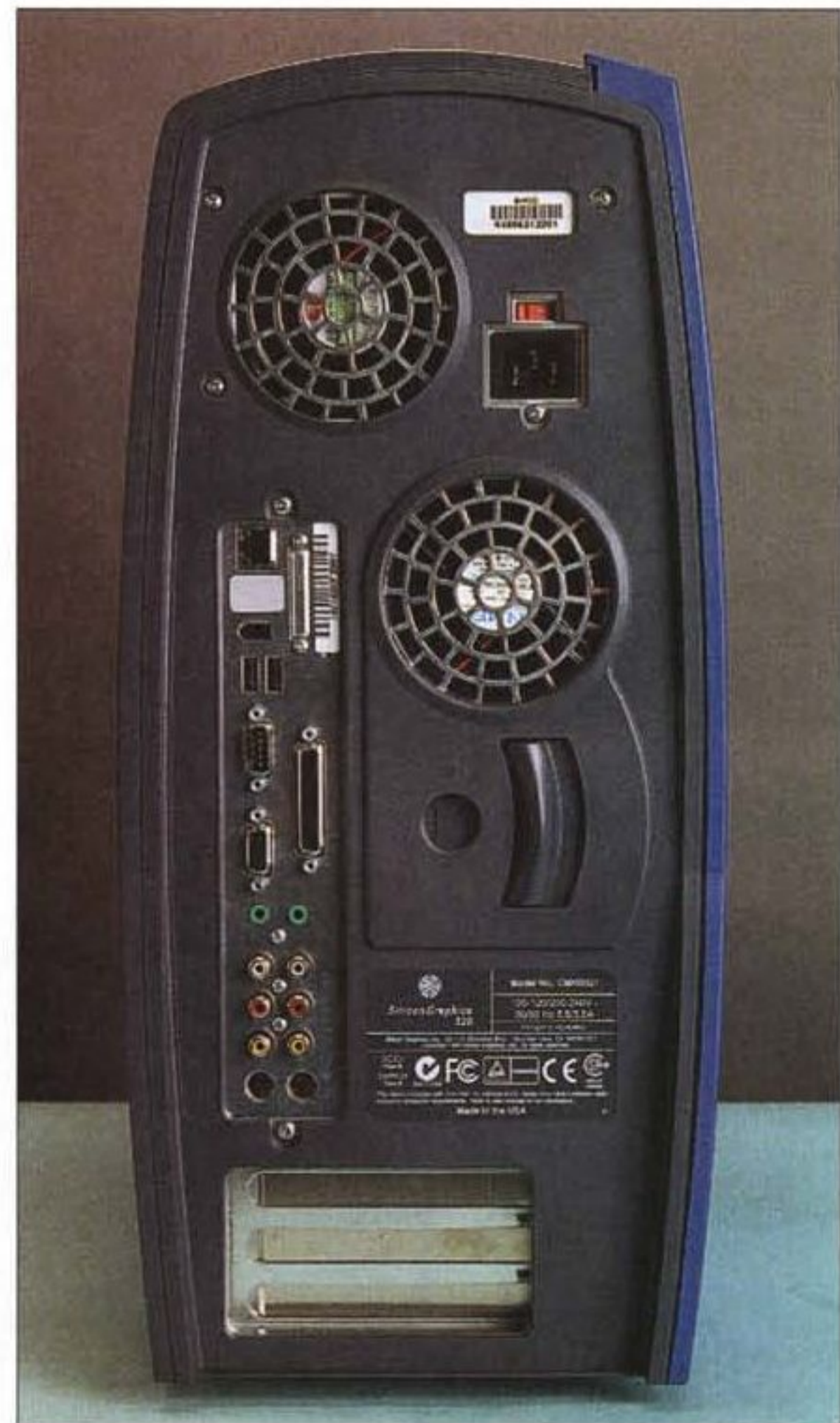
Il retro della SGI 320. Possiamo notare il completo set di connettori sulla sinistra, i tre slot PCI64 (nessuno occupato) in basso, la maniglia per lo sblocco del pannello laterale al centro, le due griglie per le ventole di aerazione e il singolo connettore per l'alimentazione.
